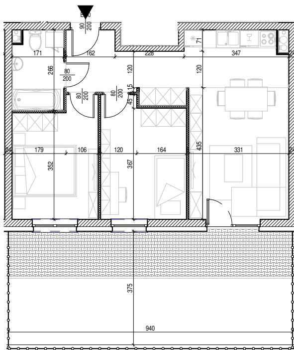
Rysunek architektoniczny
