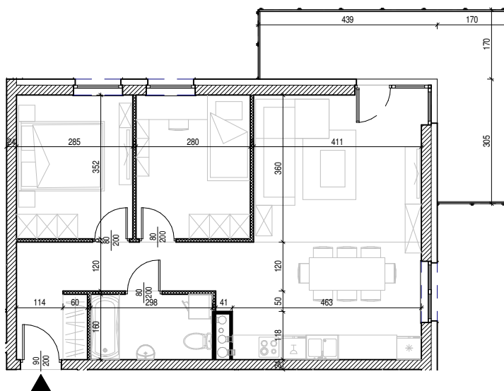
Rysunek architektoniczny
