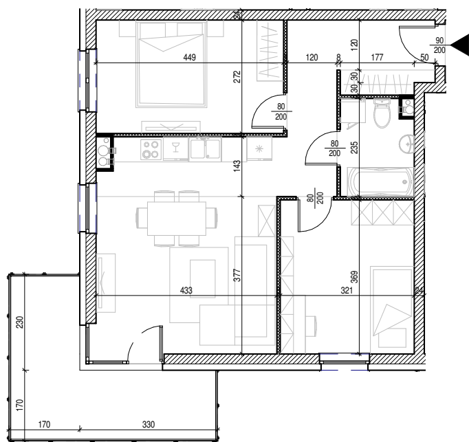
Rysunek architektoniczny
