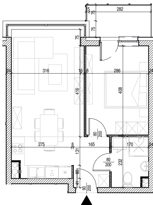
Rysunek architektoniczny
