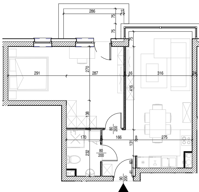
Rysunek architektoniczny
