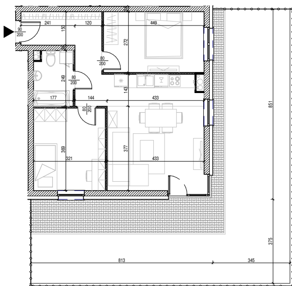
Rysunek architektoniczny
