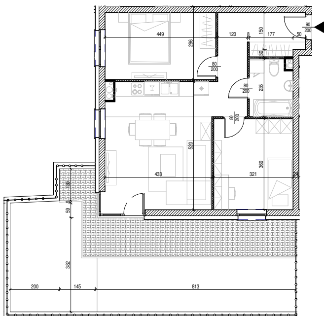
Rysunek architektoniczny
