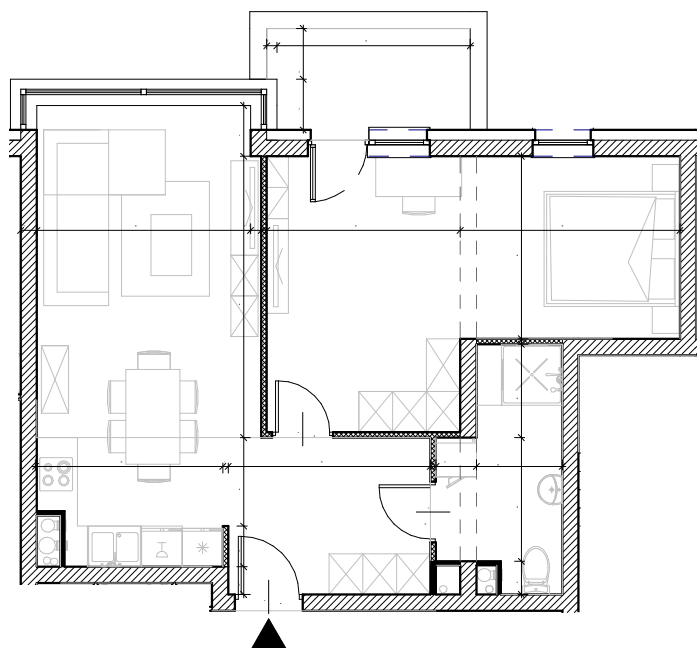
Rysunek architektoniczny
